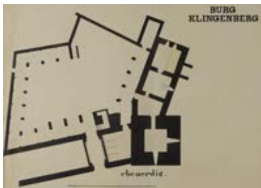
Obr. 6. Zvíkov, hrad, půdorys přízemí paláce, Antonín Šiman (?), kolem 1845–1853, zdroj: SOA Třeboň, fond Stavební správa Orlík, inv. č. 336, plán č. 439
