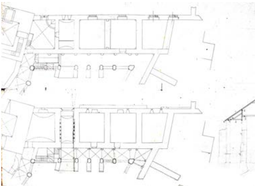
Obr. 19. Zvíkov, hrad, půdorysy přízemí a patra západního křídla paláce, Raimund Marchetti (?), před listopadem 1884, zdroj: SOA Třeboň, fond Stavební správa Orlík, inv. č. 418, plán č. 603
