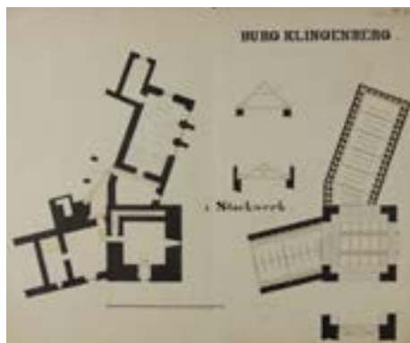
Obr. 7. Zvíkov, hrad, půdorys patra jihozápadní části paláce, Antonín Šiman (?), kolem 1845–1853, zdroj: SOA Třeboň, fond Stavební správa Orlík, inv. č. 336, plán č. 438
