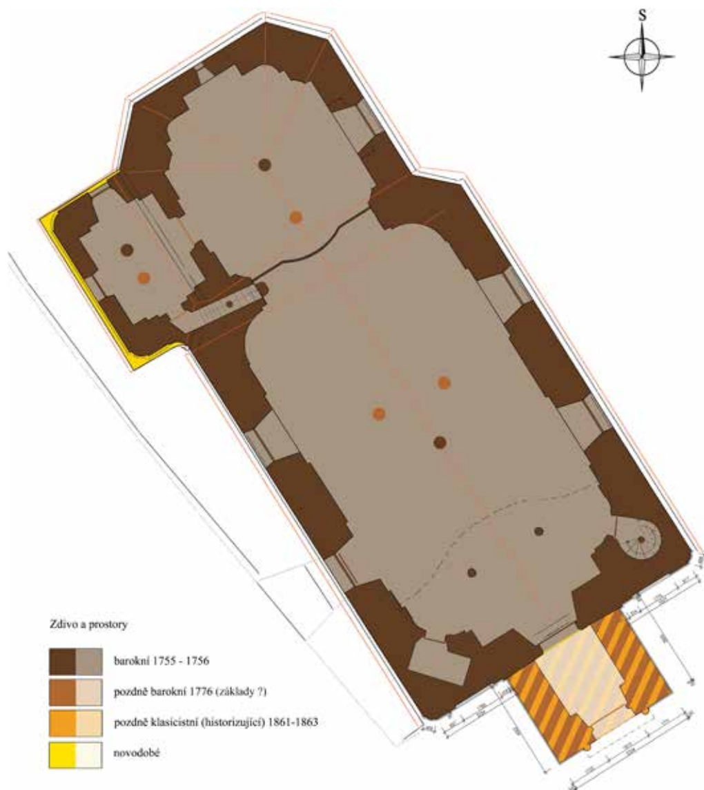
Obr. 20. Radošov, kostel sv. Václava, stavebněhistorické vyhodnocení, zdroj: Lubomír Zeman, 2019
