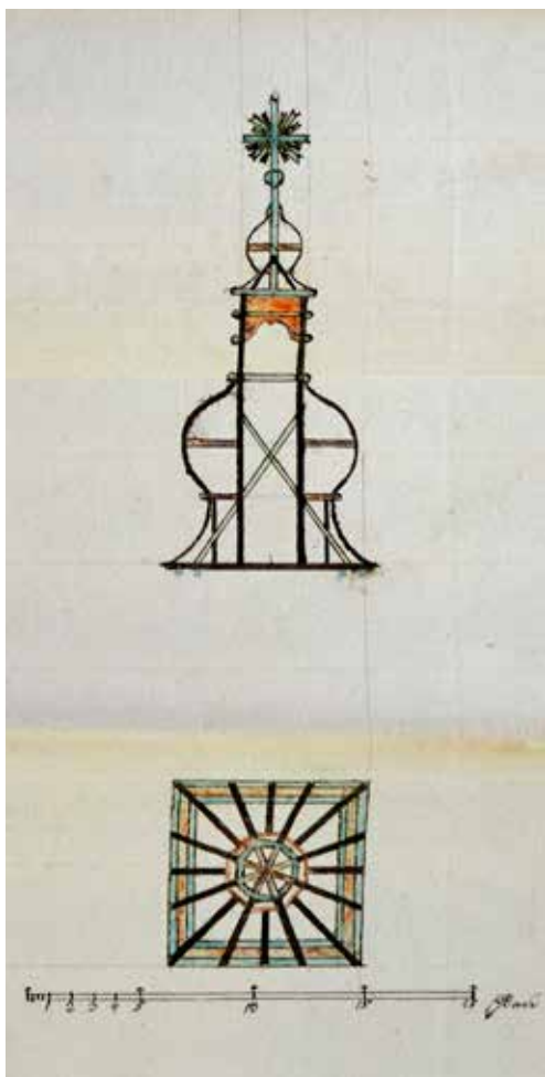
Obr. 5. Radošov, nerealizovaný návrh věže kostela sv. Václava, vazba krovu věžní bání v pohledu a půdorysu, grafické měřítko (loketní), Martin Henl (?), 1776, zdroj: SOA Plzeň, fond Vrchní úřad Ostrov, kart. 161, sign. I K2, inv. č. 57, č. 460 ½
