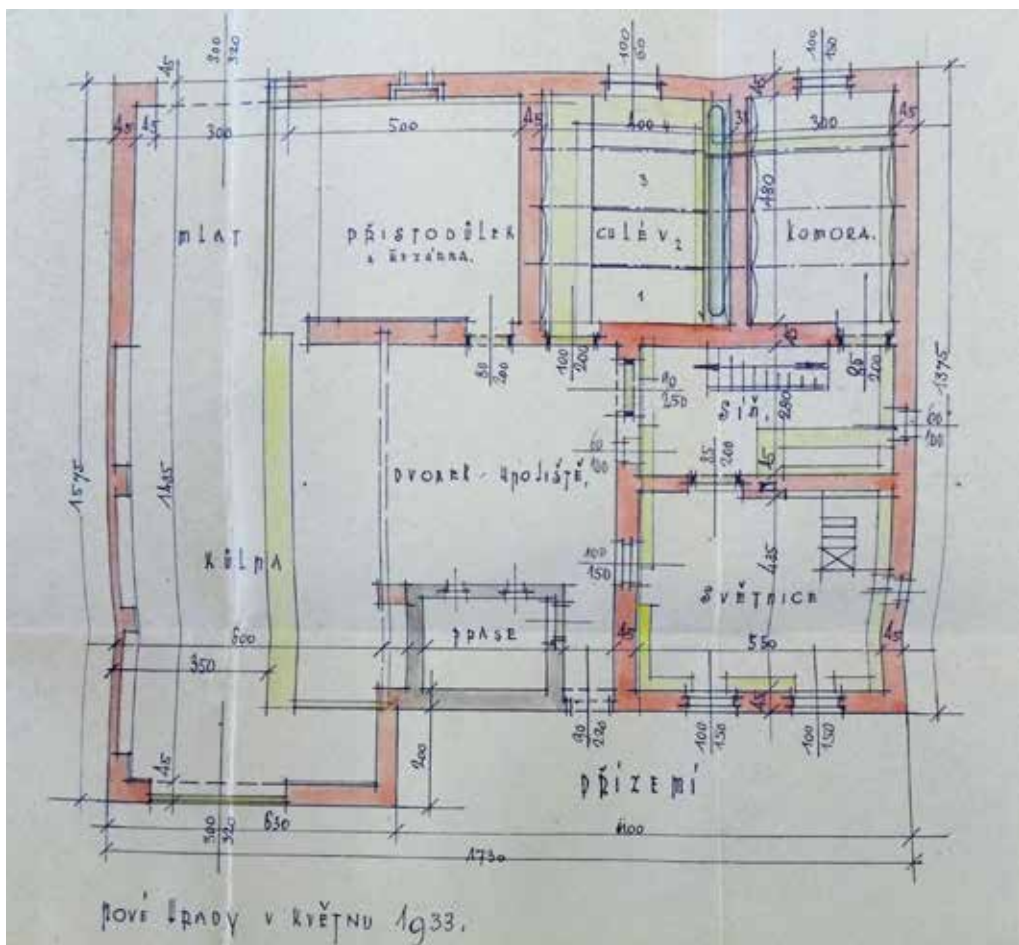
Obr. 5. Výřez ze stavebního plánu přestavby usedlosti čp. 18 z roku 1933, kreslil J. Šantrůček, Nové Hradky; plán zachycuje starší odstraňovanou stavbu, která představuje roubenou usedlost s kolmým zděným hospodářským křídlem, složeným z přístodůlku a chlévu, který je situovaný v kolmém traktu na třetí díl domu a zasahuje do podélné dispozice domu a tím zmenšuje prostor komory; ve starší situaci je zde zachycen objekt, který ve vesnici představuje typické půdorysné a materiálové řešení většiny usedlostí, zdroj: SOKA, Ústí nad Orlicí, AO Javorník, kart. č. 1, nefol.
