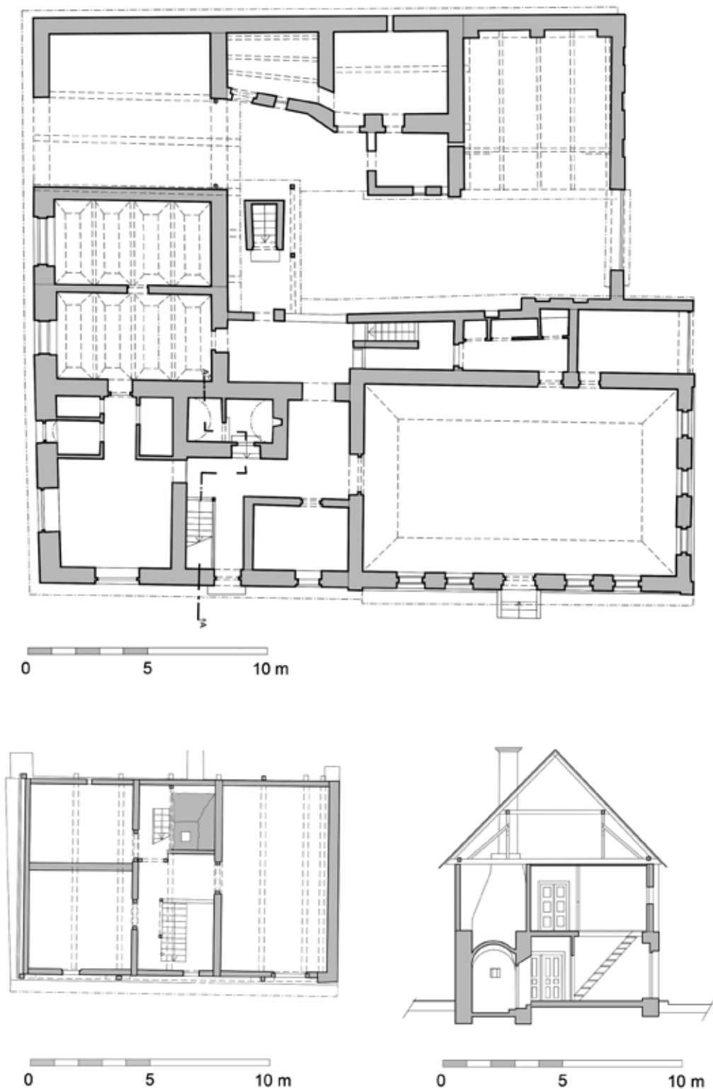
Obr. 10. Vysoká čp. 1, zaměření usedlosti, patro, přízemí, kolmý řez patrovou částí domu, zaměření: J. Svobodová, J. Pochmanová, autor: Jitka Svobodová, 2022
