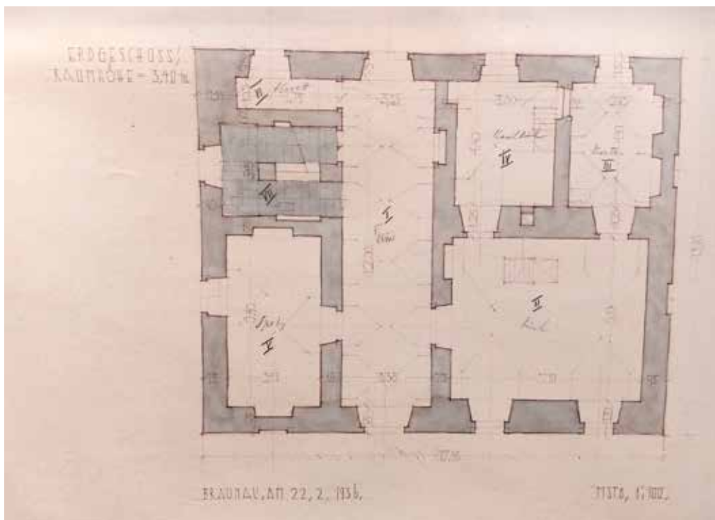
Obr. 5. Půdorys přízemí fary na skice F. J. Wilda z 22. 2. 1936, zdroj: Státní oblastní archiv Hradec Králové, Velkostatek Broumov, kart. 450, inv. č. 2288, Správa velkostatku 1929–1944
