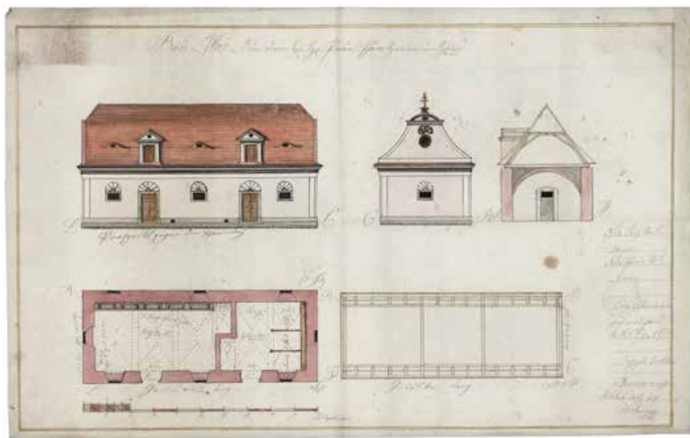
Obr. 3. Plán maštale pro farní dvůr v Šonově z 27. 2. 1825, zdroj: Státní oblastní archiv Hradec Králové, VS Broumov, inv. č. 7380
