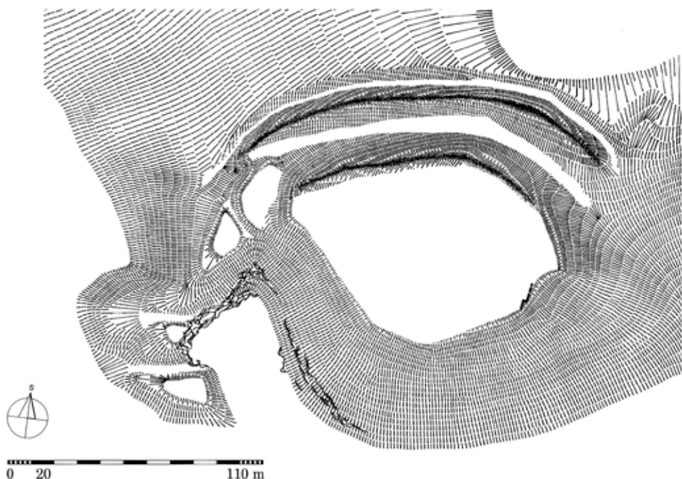
Obr. 3. Půdorysné zaměření hradního návrší Landeku s dochovaným zbytkem zdi (vyznačeno černě), převzato z: KOUŘIL, Pavel – PRIX, Dalibor – WIHODA, Martin, Hrady českého Slezska , s. 247, obr. 160
