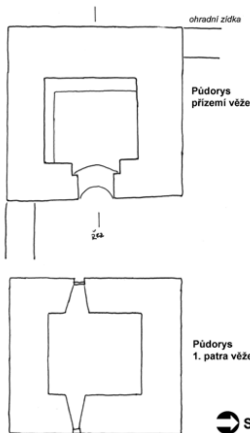
Obr. 7. Prosetín, areál kostela sv. Markéty, samostatně stojící zvonice, kresebná dokumentace věže, půdorys a řez, zaměření a kresba: autor
