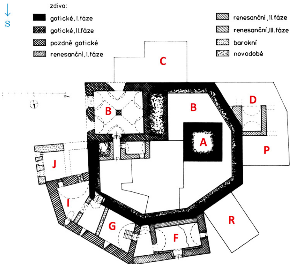
Obr. 18. Pasovary, bývalá tvrz, půdorys sklepů, Michael Rykl, 1985
