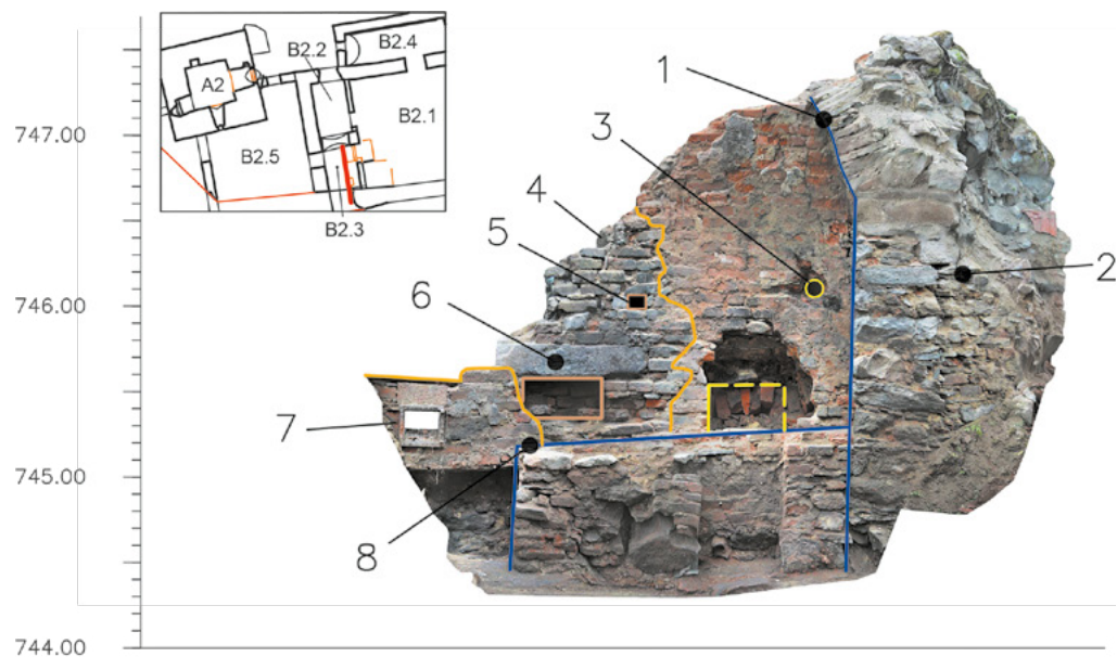
Obr. 23. Pasovary, bývalá tvrz, fotoplán vnitřní východní stěny černé kuchyně místnosti B2.3 s vyznačením nálezů, fotoplán: GEO-CZ, s. r. o., 2019, zákres Daniel Šnejd, 2023. Legenda: 1 – náběh renesančního klenebního pasu, 2 – líc špalety vstupu do jižní přístavby, 3 – kruhový sopouch odvodu kouře z pece, 4 – torzo kouřovodu zaniklých kamen provedené z cihel, 5 – čtvercový sopouch staršího topeniště, 6 – překlad nad příkladacím otvorem zaniklých kamen z druhotně použitého gotického ostění, 7 – konstrukce novodobého sporáku z 1. pol. 20. stol. s příkladacím otvorem otočeným do černé kuchyně, 8 – nároží zvýšené podesty pro vaření před ústím topenišť. Modrá – renesanční, hnědá – barokní, žlutá – přelom 19. a 20. století
