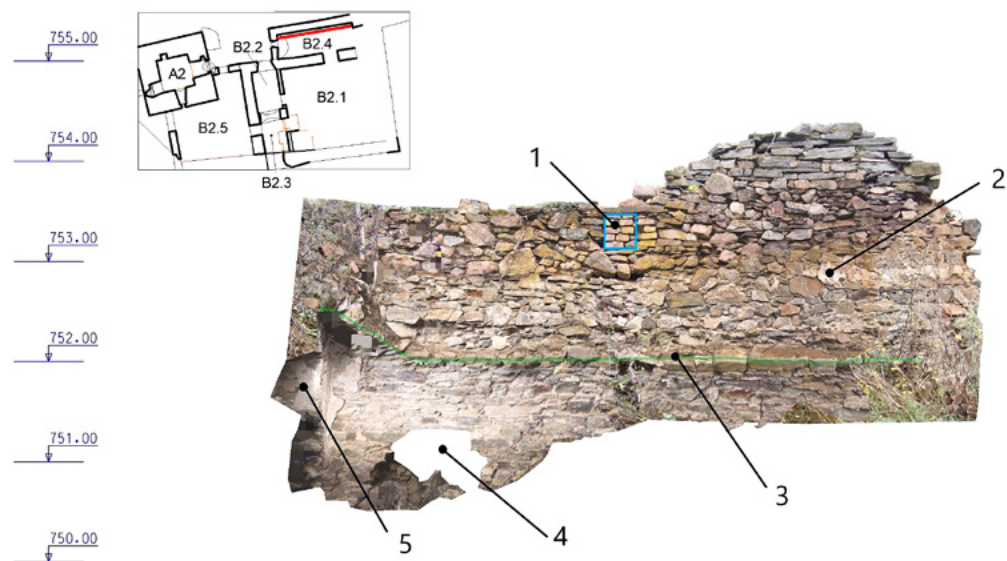
Obr. 26. Pasovary, bývalá tvrz, fotoplán vnitřní severní stěny místnosti B2.4 s vyznačením nálezů, foto-plán: GEO-CZ, s. r. o., 2019, zákres Daniel Šnejd, 2023. Legenda: 1 – kapsa po trámu v úrovni odsoků pro uložení stropu sousední síně, 2 – fragment omítky, dochovaný v úrovni klenebního zasypu, 3 – torzo nábehu valené klenby, 4 – místo okenní niky, 5 – špaleta druhého okna otočeného ke vstupu do paláce. Modrá – renesanční, zelená – 19. století
