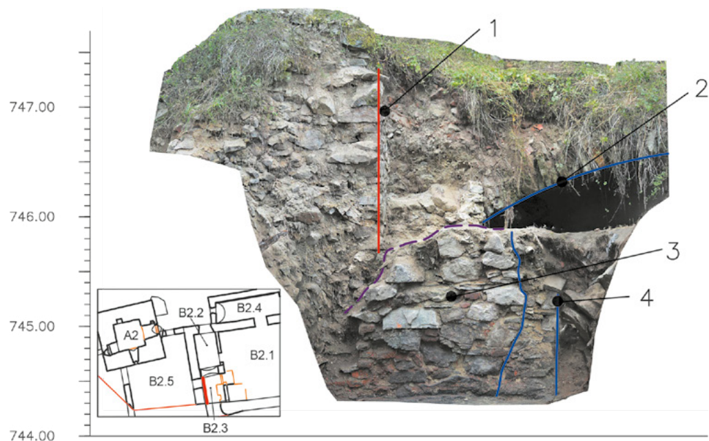
Obr. 24. Pasovary, bývalá tvrz, fotoplán vnitřní západní stěny černé kuchyně místnosti B2.3 s vyznačením nálezů, fotoplán: GEO-CZ, s. r. o., 2019, zákres Daniel Šnejd, 2023. Legenda: 1 – vnitřní líc obvodové gotické hradby, 2 – klenba sklepa renesančního paláce, 3 – vnitřní líc obvodového zdiva gotického paláce, 4 – špaleta vstupu z černé kuchyně do sklepa renesančního paláce. Červená – 14. století, fialová – 15. století, modrá – 16. století
