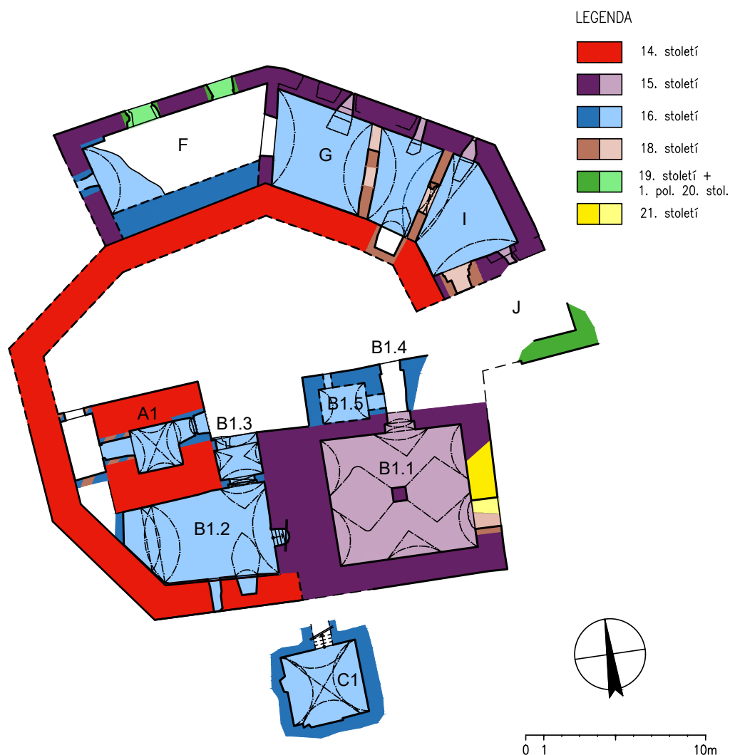
Obr. 19. Pasovary, bývalá tvrz, půdorys sklepů s vyhodnocením stáří konstrukcí. Geodetické zaměření: CePT, s.r.o., 2019, vyhodnocení: Daniel Šnejd, 2023
