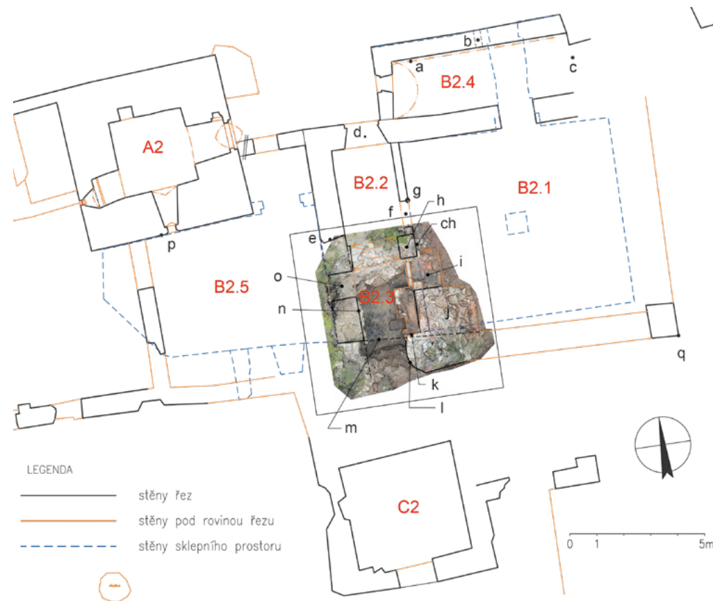
Obr. 22. Pasovary, bývalá tvrz, půdorys prvního patra, výřez obytné části tvrze s věží, vložen fotoplán černé kuchyně, GEO-CZ, s. r. o., 2019, zákres: Daniel Šnejd, 2023. Legenda: B2.1 – světnice, B2.2 – vstupní síň, B2.3 – černá kuchyně (příkladací prostor), B2.4 – severní renesanční přístavba, B2.5 – prostor renesanční klenuté místnosti s nástěnnou malbou, A2 – věž, C2 – jižní renesanční přístavba; a – fragment valené klenby, b – kapsa po trámu, c – dveřní či okenní nika s dochovanou levou špaletou, d – vstup do gotického paláce z nádvoří, e – špaleta vstupu z gotického paláce do místnosti B2.5, f – vstup ze síně do světnice, g – fragment zárubně se závěsem barokního typu, h – střední pilíř dvojité slepé arkády oddávající síň s kuchyní od světnice, ch – zazděný osvětlovací krb, i – torzo sporáku s příkládáním z černé kuchyně, j – torzo pece, k – náběh klenutí arkády, l – zaoblená špaleta vstupu ze starého paláce do jižní přístavby C2, m – hypotetický průběh hradby pod úrovní podlahy černé kuchyně, n – vnitřní líc obvodové zdi gotického paláce, o – v renesanci proražený vstup do sklepa pod místností B2.5, p – místo nástěnné malby před jejím transferem, q – v úrovni přízemí se dochoval pouze fragment nároží gotického paláce, l – renesanční okno stejného typu jako u objektu F, popis: Daniel Šnejd, 2023, foto: Veronika Babická, 2019
