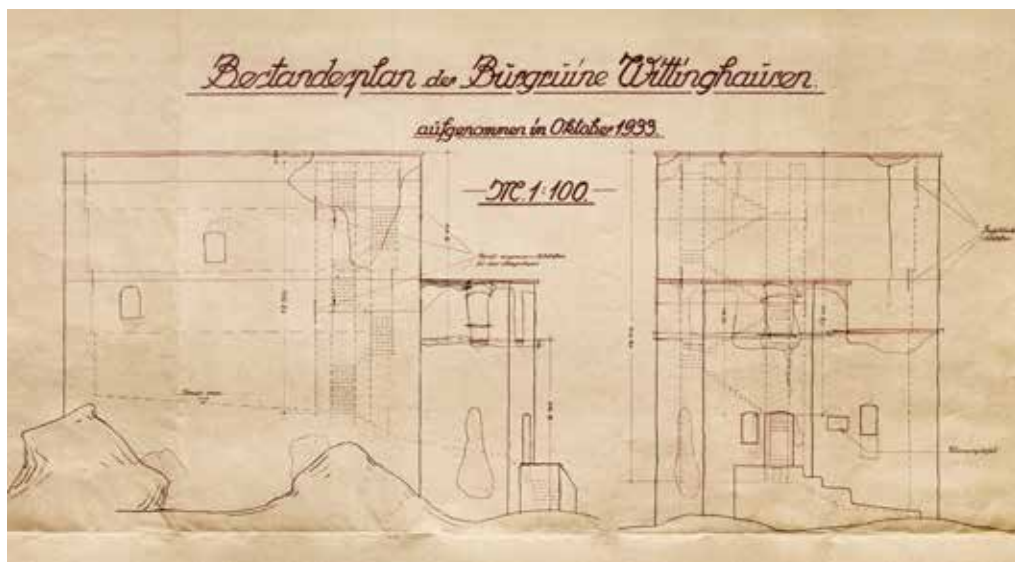
Obr. 7. Vítkův Kámen, plán stavebních oprav, 1933, zdroj: SOA v Třeboni, odd. Český Krumlov, fond Schwarzenberská ústřední stavební správa České Budějovice, dílčí inventář stavebních plánů 1773–1944, inv. č. 2281
