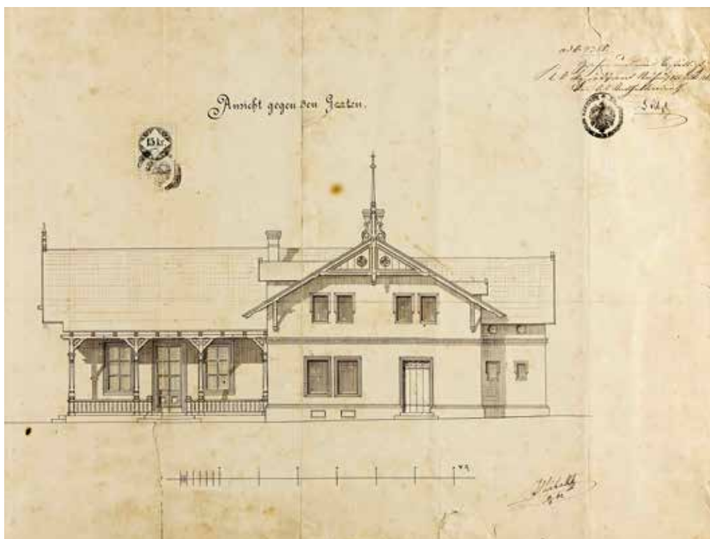
Obr. 1 a 2. Jindřichův Hradec, výletní restaurace Rudolfov, průčelí a boční fasáda, stavební výkresy Josefa Zítka, 1862, zdroj: SOA v Třeboni, odd. Jindřichův Hradec, Vs Jindřichův Hradec, inv. č. 5337
