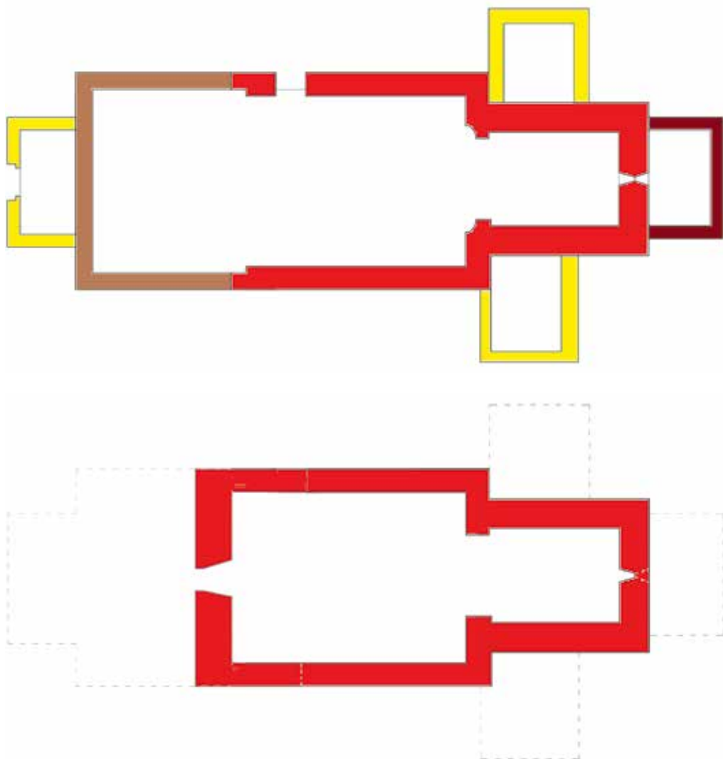
Obr. 8. Štěpánov nad Svratkou, kostel. Nahoře zjednodušený půdorys kostela v úrovni vstupu s rozlišenými etapami stavebního vývoje: červeně gotické zdivo, světle hnědou raně barokní prodloužení lodě, tmavě hnědou přístavba sakristie, žlutě konstrukce z dvacátých let 20. století. Dole rekonstrukce původní dispozice kostela z období druhé poloviny 13. století, zaměření a kresba: autor
