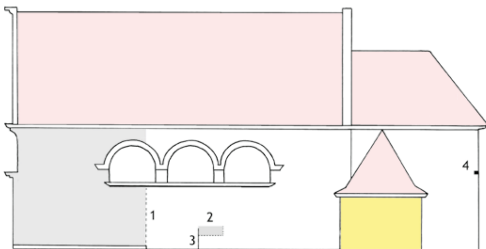
Obr. 15. Štěpánov nad Svratkou, kostel. Nahoře pohled na severní stranu lodi v době obnovy vnějších omítek, foto: autor, 2020. Dole schematická skica objevených spár na jižní straně (kresba autor): 1 – spára mezi původní částí lodi a jejím barokním prodloužením (vyneseno šedou barvou); 2 – hypotetický pozůstatek barokního okna; 3 – spára interpretovaná jako započatý jižní vstup; 4 – kamenná konzola pod patou východního štítu kněžiště. Žlutě zvýrazněna novodobá sakristie
