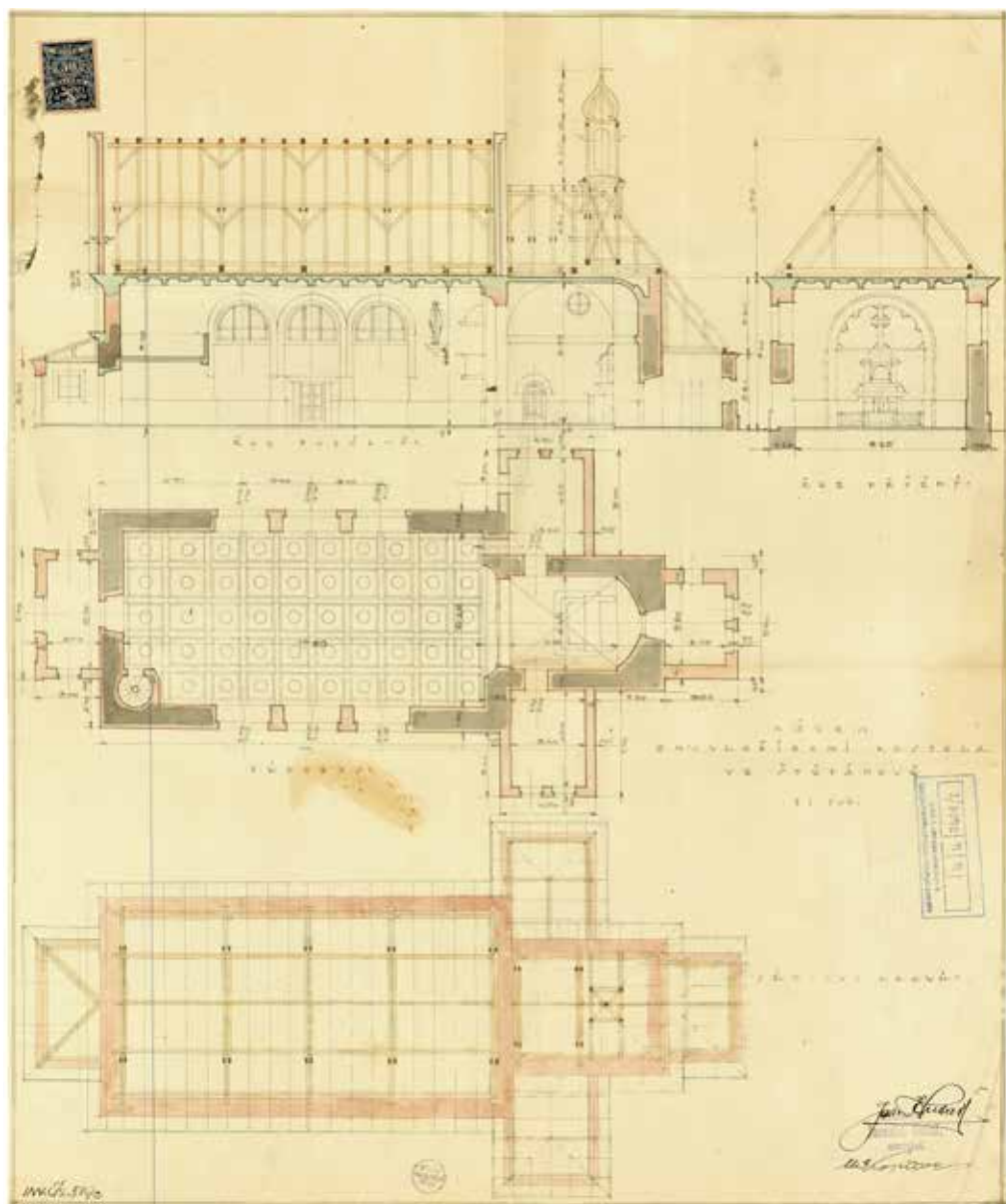
Obr. 5b. Plánová dokumentace na obnovu vyhořelého kostela z roku 1917 (nerealizováno) a mladší, patrně z roku 1923, která již odpovídá současnému stavu kostela, zdroj: archiv NPÚ, ÚOP v Telči, inv. č. 7408
