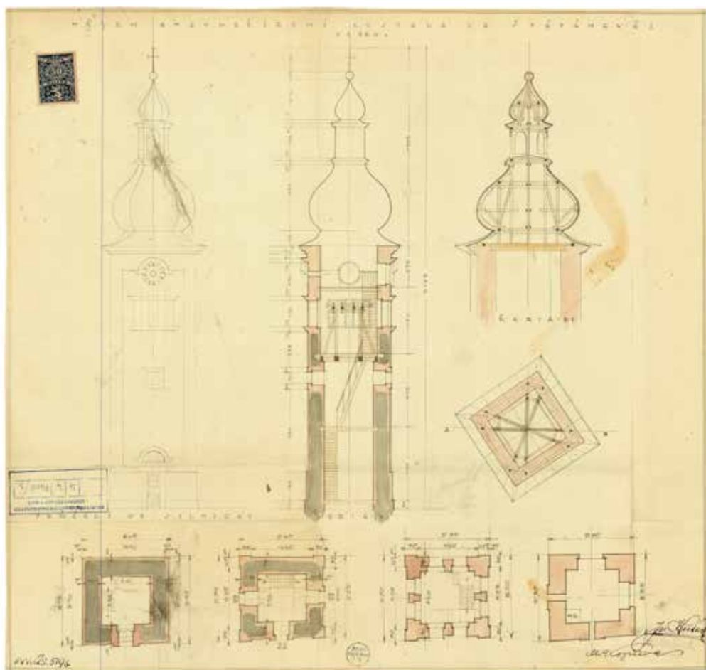
Obr. 5c. Plánová dokumentace na obnovu vyhořelého kostela z roku 1917 (nerealizováno) a mladší, patrně z roku 1923, která již odpovídá současnému stavu kostela, zdroj: archiv NPÚ, ÚOP v Telči, inv. č. 7408
