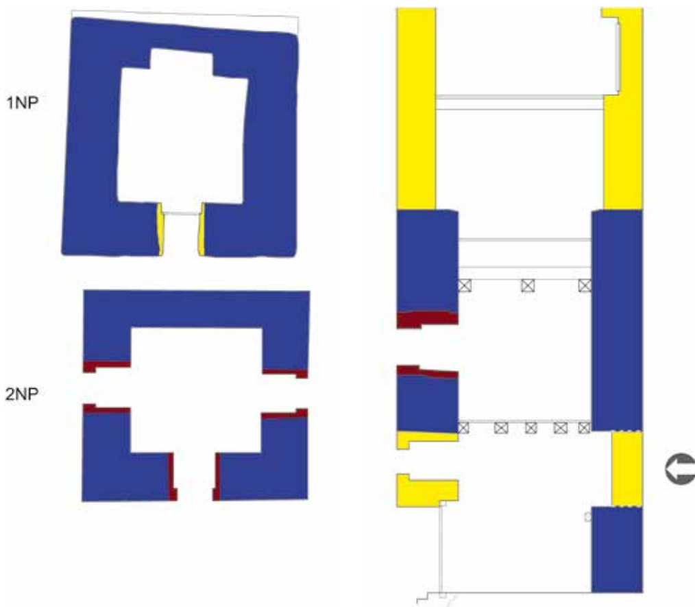
Obr. 20. Štěpánov nad Svratkou, věž. Stavební vývoj zvonice: modře konstrukce ze 16. století, tmavě hnědou z doby okolo poloviny 18. století, žlutě novodobě z dvacátých let 20. století (zaměření a kresba: autor). Vlevo půdorys přízemí a prvního patra. Vpravo řez S–J, šipkou označen původní vstup do věže, pod ním se nachází pozůstatek zazděného dendrochronologicky datovaného trámu
