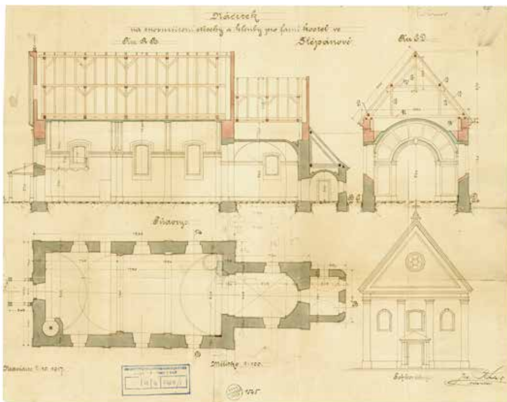
Obr. 5a. Plánová dokumentace na obnovu vyhořelého kostela z roku 1917 (nerealizováno) a mladší, patrně z roku 1923, která již odpovídá současnému stavu kostela, zdroj: archiv NPÚ, ÚOP v Telči, inv. č. 7408
